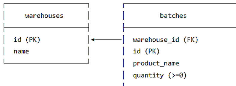
Рисунок 1 – ER-диаграмма
