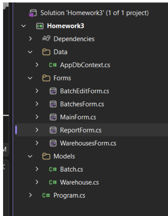
Рисунок 2 Архитектура приложения
